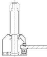
(für Montage innen Beschattung, ohne Oberlicht)
